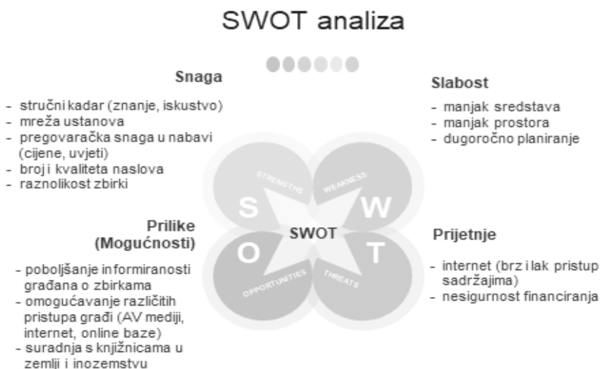
Slika 2. SWOT-analiza
