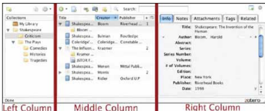
Slika 1. Zotero panel
